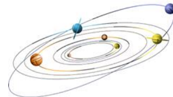
Système solaire
