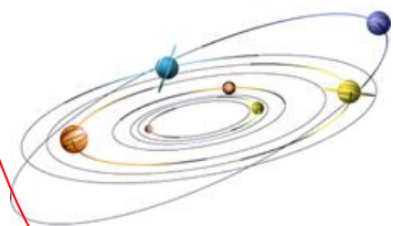
Système solaire
